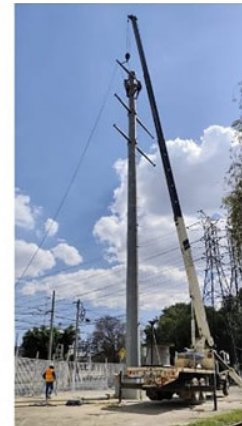
Obra civil poste tronco cónico conformada por una pila de 12 m de profundidad y dado de cimentación Trabajo realizado en diciembre de 2024
